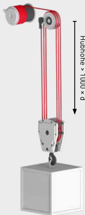
Heben einer ungeführten Last mit mehrerer Seilsträngen bei Hubhöhen größer als 1000 \times \text{Seildurchmesser}
