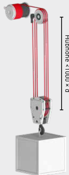
Heben von ungeführten Lasten mit mehreren Seilsträngen und Hubhöhen kleiner 1000 \times d
