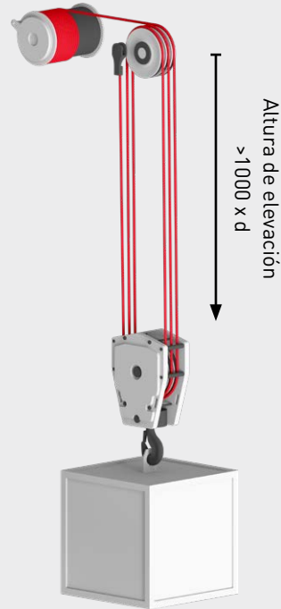
Izado de una carga sin guiado en varios ramales a una altura de elevación superior a 1000 x el diámetro del cable
