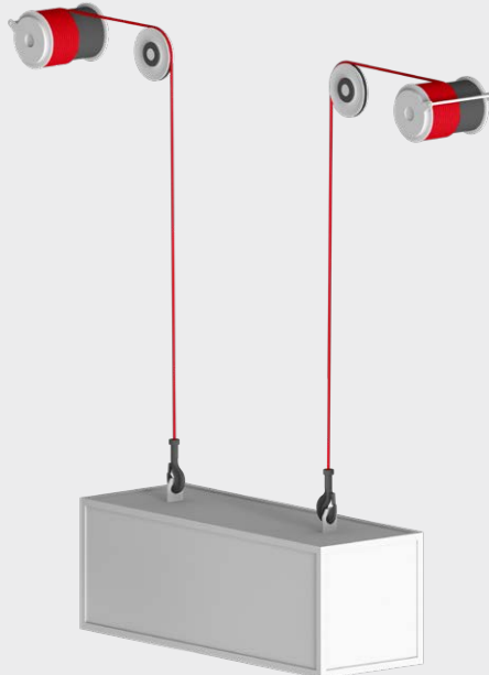
Izado de una carga sin guía con cables a derechas e izquierdas que operan en pareja
