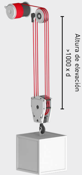
Izado de una carga sin guía en varios ramales a una altura de elevación de hasta 1000 x diámetro del cable
